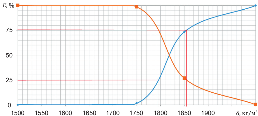
Рис. 1. Кривые разделения Тромпа: 1 – порода; 2 – концентрат; E – извлечение, \delta – плотность разделения.
