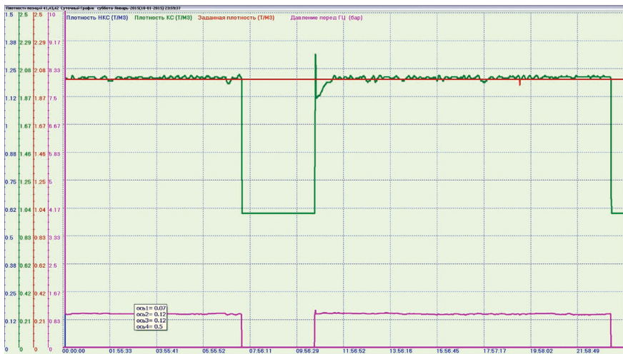
Рис. 3. График поддержания плотности кондиционной суспензии (работа в автоматическом режиме).
